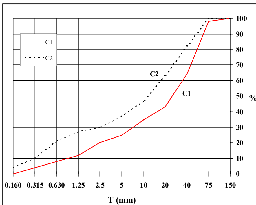
Fig. 16: Curva granulométrica recomendada para áridos tamaño máximo de 76,2 mm (McIntosh)
