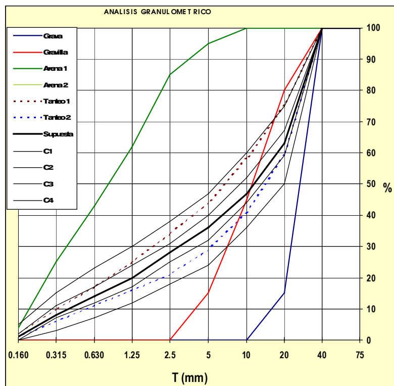
Fig. 18: Ejemplo proporcionamiento de áridos por tanteo
