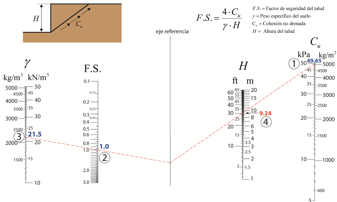
Nomograma para el cálculo de la altura crítica de un suelo cohesivo a corto plazo
