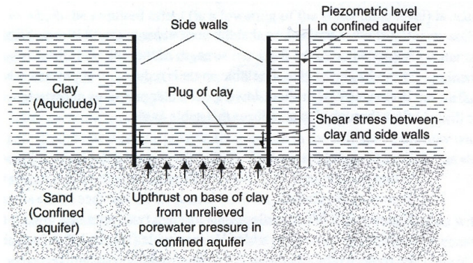
Figura 2.- Levantamiento del fondo debido a la excavación en un suelo de baja permeabilidad sobre un acuífero confinado, en recinto delimitado por diafragma (PREENE et al., 2004).
