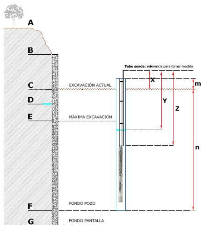
Figura 11.- Esquema sección y cotas de interés de cada pozos.
