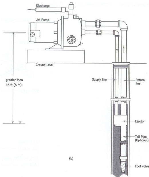
Figura 6.- Cuerpo eyector en la instalación de interior del pozo
