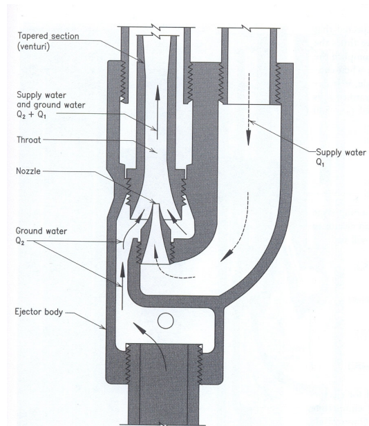
Figura 7.- Cuerpo eyector
