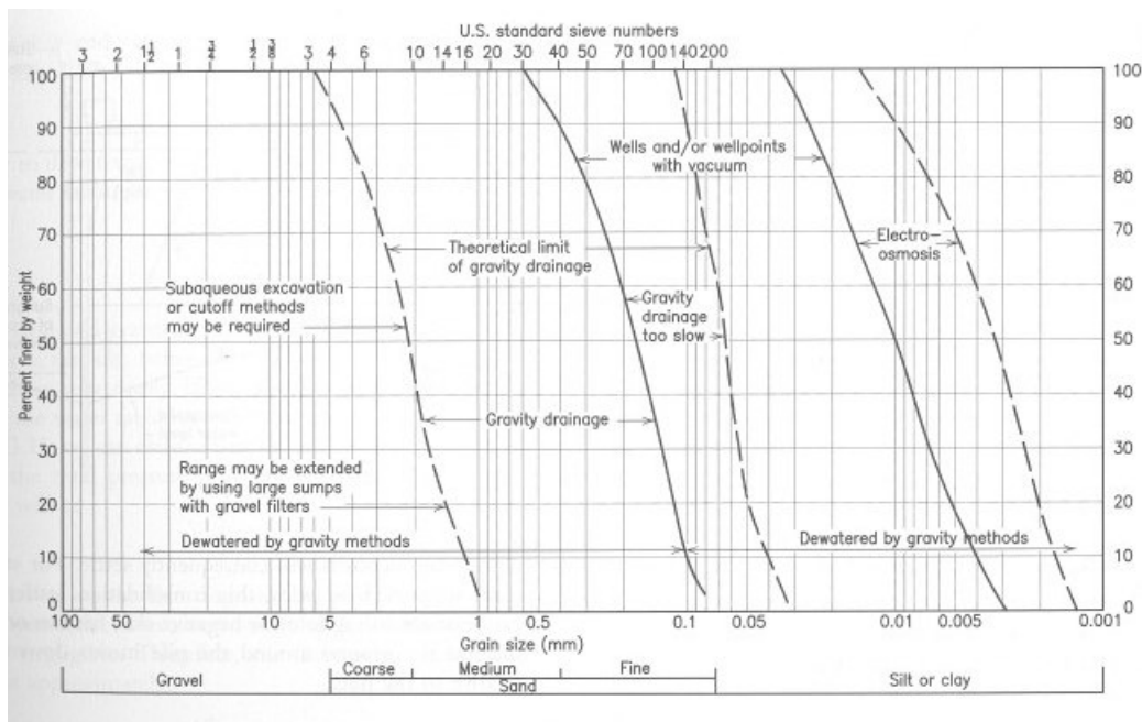
Figura 8.- Sistemas de drenaje aplicables a diferentes tipos de suelos (POWERS et al., 2007; pg 45)
