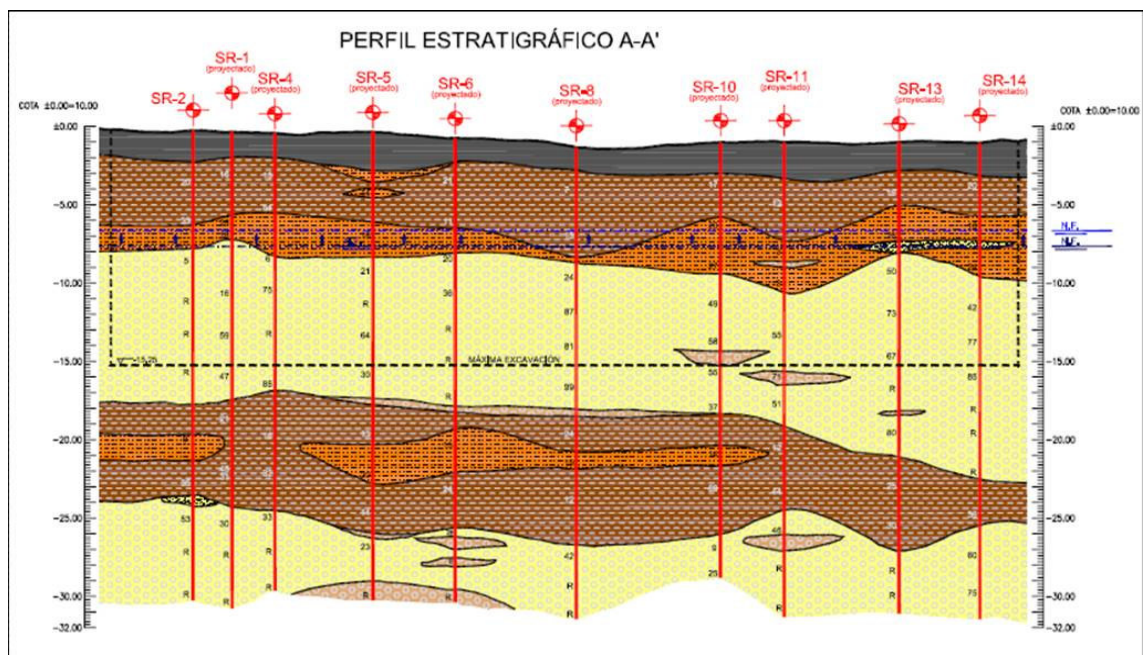
Figura 9.- Perfil geotécnico de la parcela
