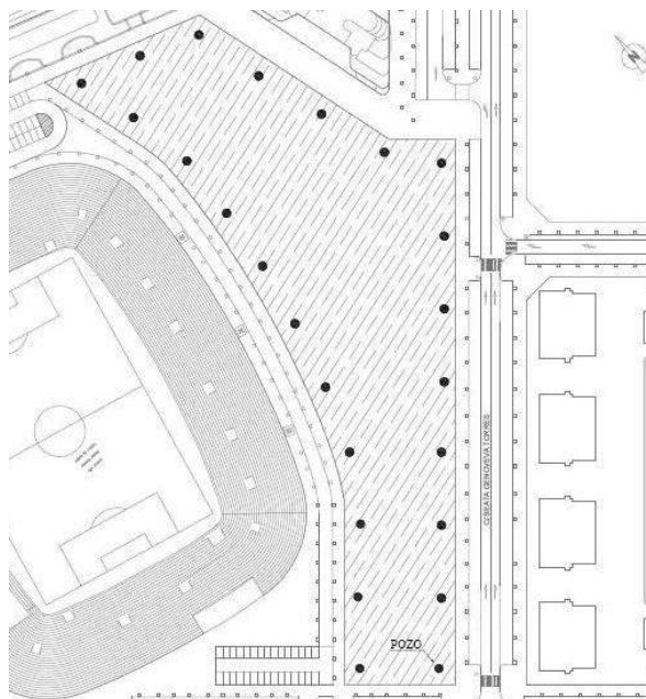
Figura 10.- Esquema de la ubicación de los pozos en el interior de la parcela objeto de actuación.
