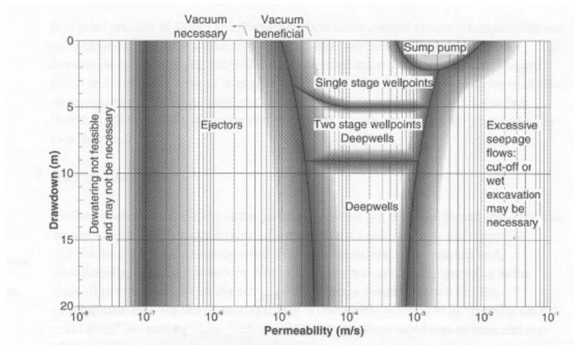
Figura 5.- Rango de aplicación de las técnicas de bombeo recomendables para controlar las aguas subterráneas. (PREENE, et al., 2004).
