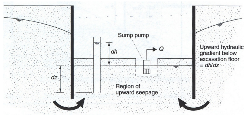
Figura 4.- Esquema sobre el riesgo de sifonamiento (PREENE et al., 2004).
