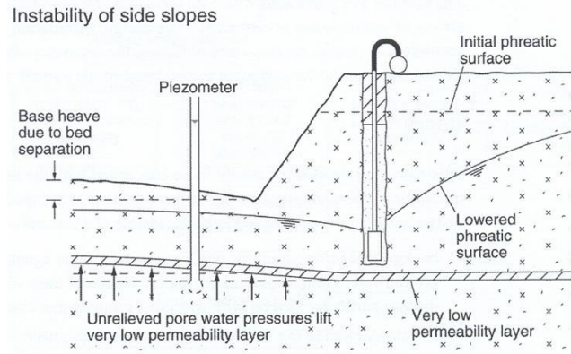
Figura 3.- Levantamiento del fondo debido a la excavación en un suelo sobre un acuífero confinado, en recinto no delimitado por diafragma (PREENE et al., 2004).
