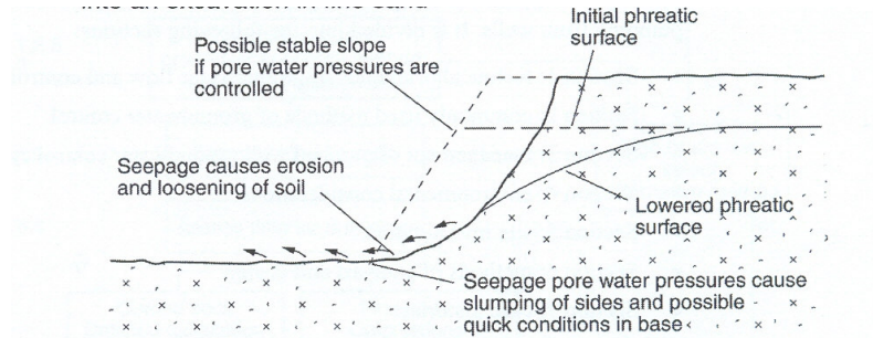
Figura 1.- Esquema del deslizamiento de un talud (PREENE, et al., 2004)
