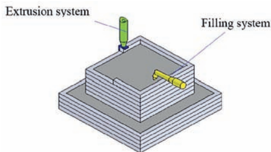
Figura 2. Sistema automático de construcción Contour Crafting.
