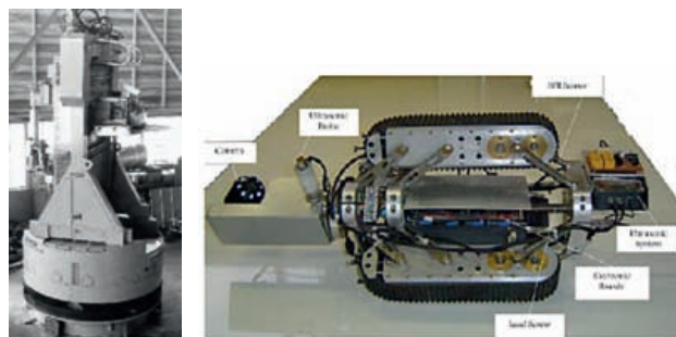
Figura 2 (izquierda). Robot para demolición de centrales nucleares.
