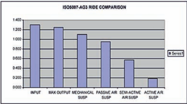
Figura 3. FRF y aceleración ISO5007 con distintos tipos de suspensión.
