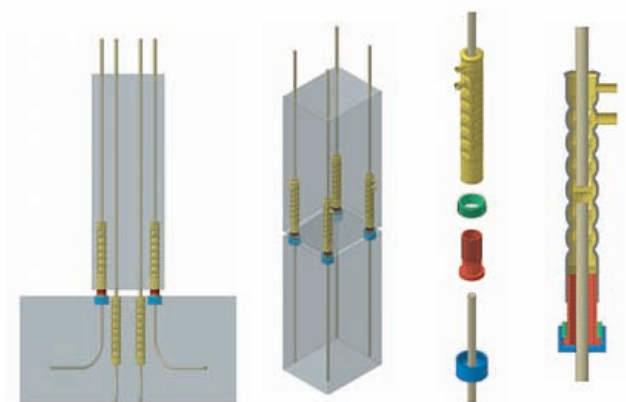
Figura 5: Nuevo sistema de unión de elementos prefabricados para resolver la hiperestaticidad de uniones, que consigue eliminar la excentricidad de esfuerzos y consigue resultados antisísmicos óptimos. Fuente: B.S. Italia.
