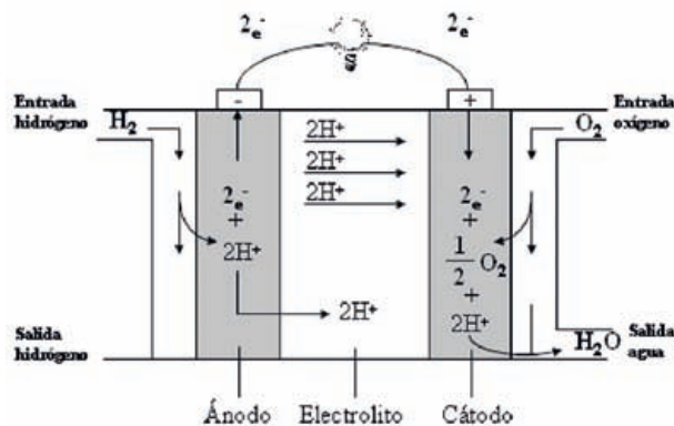
Figura 4. Sistema de almacenamiento de energía. Pila de combustible.
