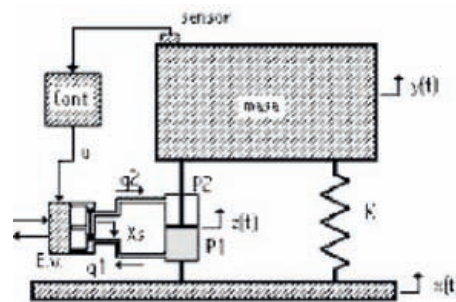
Figura 2. Modelo de simulación de un sistema activo de reducción de vibraciones.
