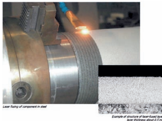
Figura 1. Ejemplo de aplicación de tratamiento superficial por técnicas láser.
