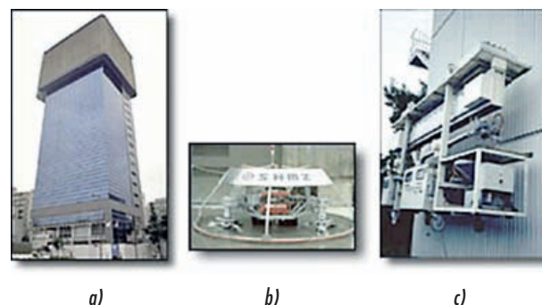
Figura 1. Tres ejemplos de automatización en la construcción. La figura a) es un edificio de construcción totalmente automatizada en Nagoya, Japón. La figura b) es un robot para el acabado de superficies de hormigón. La figura c) es un robot con movimiento vertical para pintar fachadas.
