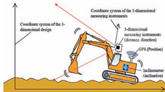
Figura 5. Robotización de una excavadora incorporando sensores en las articulaciones, medidas -D, inclinómetros y sistemas GPS.
