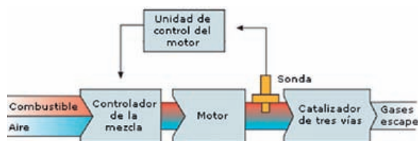
Figura 3. Sistema de control de motor para reducción de emisión de gases.
