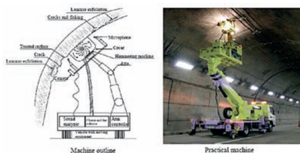
Figura 4. Robot para la reparación de paredes en túneles.
