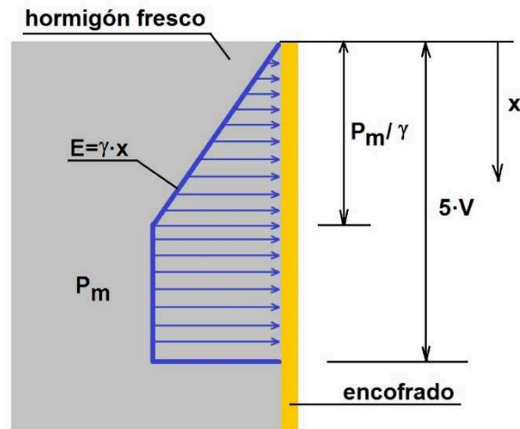
Figura 3. Empuje del hormigón fresco según norma DIN-18218
